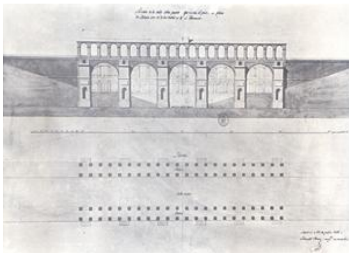
Proyecto de viaducto. Silvestre Pérez, 1810
